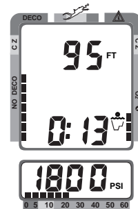
Fig. 39 - Main Display (Alt On)
