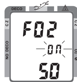
Fig. 27 - Set FO2 50% Default On/Off
