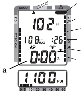
Fig. 76 - High O 2
