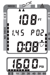
Fig. 74 - High PO 2 (= /> 1.40 ATA)
