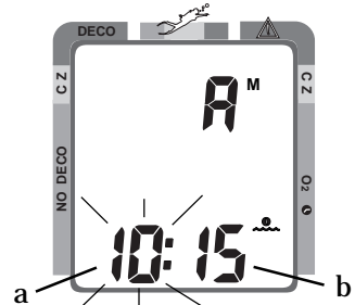
Fig. 24 - Set Time
